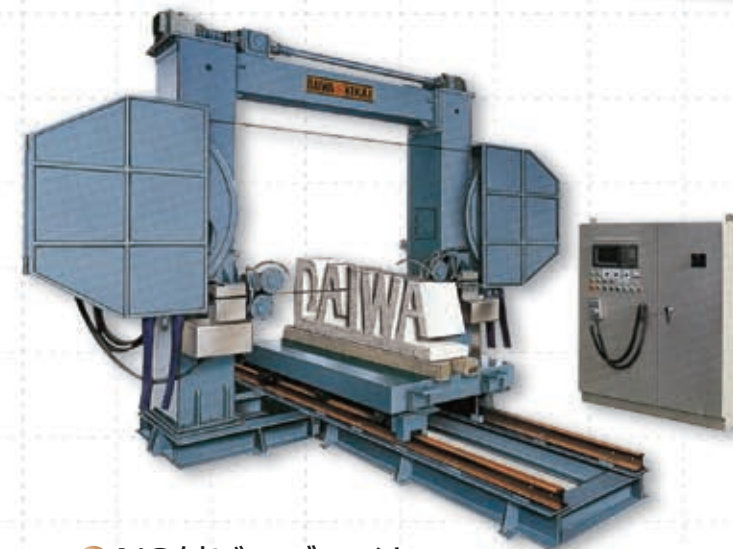
● NC付ビーズワイヤソー
